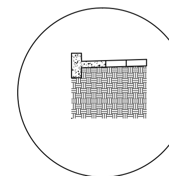
Detalhe do Meio Fio e Sarjeta.
